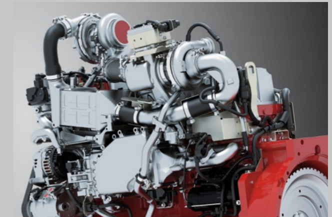
Κινητήρας Deutz 246 ίππων (181 kW): άμεση απόκριση με υψηλή ροπή εκκίνησης και σημαντική εφεδρική ροπή με έως και 5% λιγότερη κατανάλωση καυσίμου και AdBlue.
